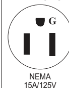
NEMA 5-15P
