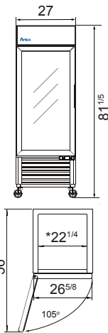
MCF8722GRL
